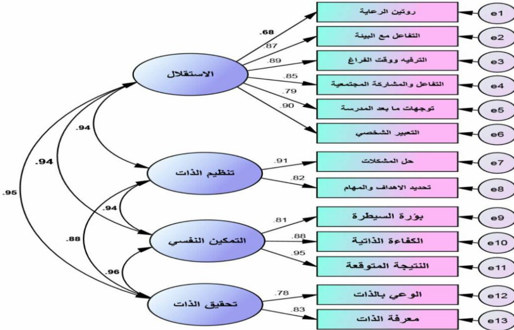
شكل (١) التحليل التوكيدي لأبعاد مقياس تقرير المصير
